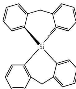
UGH4
