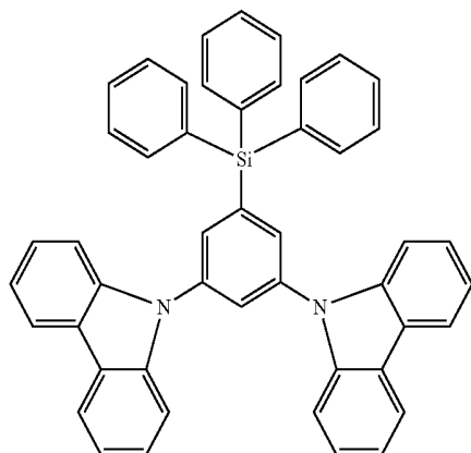
SimCP
